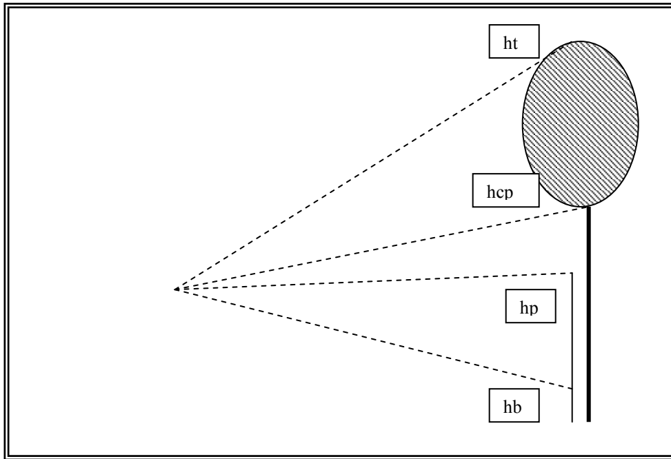
Gambar 6. Pengukuran tinggi pohon dengan clinometer
